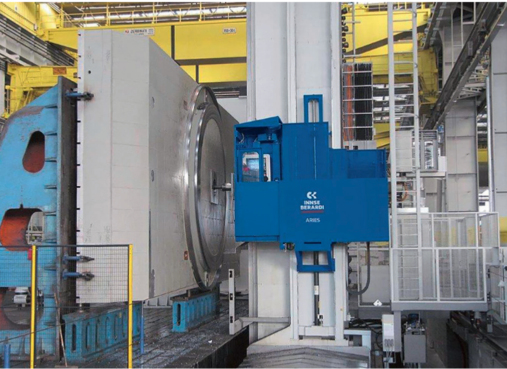
4 Horizontal-Variante ›Aries‹: Die Baureihe gibt es als Hochleistungsmaschinen mit hohem Drehmoment für die Schwerzerspannung oder als Hochgeschwindigkeitsmaschinen für Flugzeugkomponenten aus Verbundwerkstoffen © Innse-Berardi
